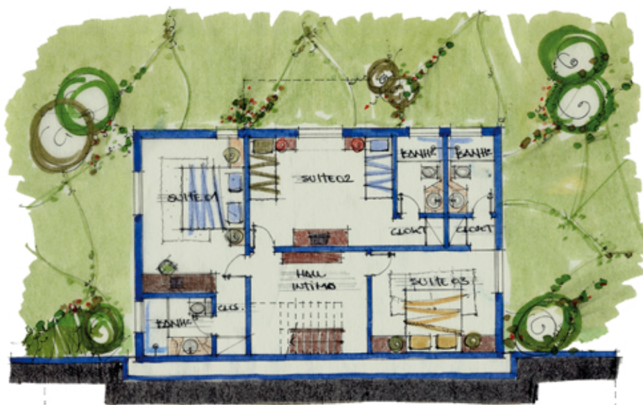
PLANTA BAIXA - NÍVEL TERRAÇO
